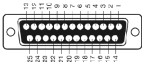
connettore porta parallela DB25F
